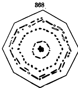
Leucite.
